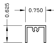
Frame Filler 999412
