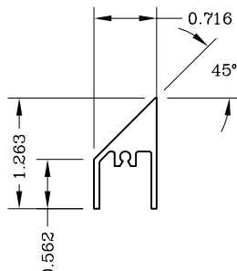
45° Beveled Filler 990883
