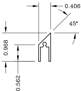
45° Beveled Filler 990763
