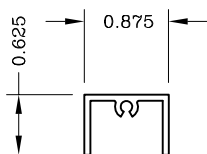
Frame Filler 999402
