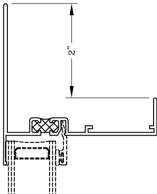
200013 Frame Head w 2” Flange
