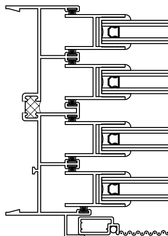
Jamb IG/IG
