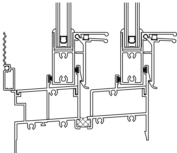
Sill IG/IG
