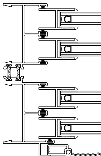
Jamb IG/IG
