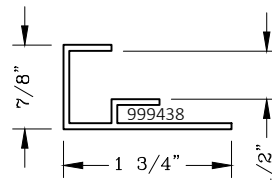
1/2" Drywall Trim
