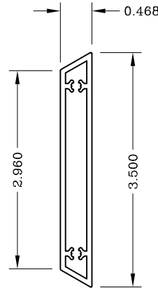
Trapezoidal 670092
