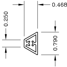
Trapezoidal 670090
