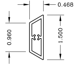
Trapezoidal 670094
