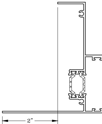
2" Flange Frame Jamb P/N 020402
