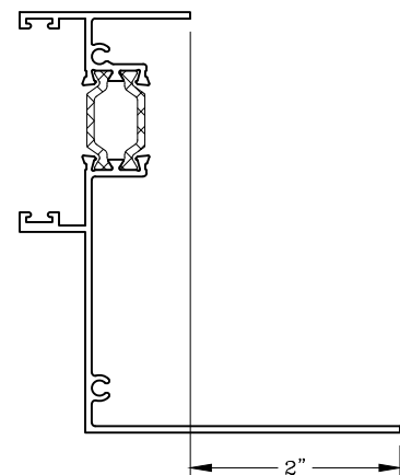
2" Flange Frame Jamb P/N 020403
