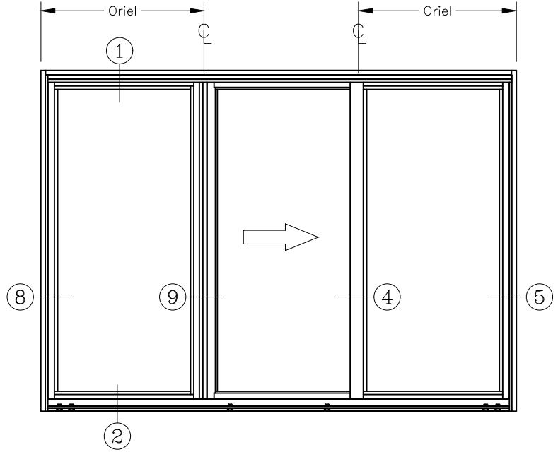
ELEVATION XOX - Shown
