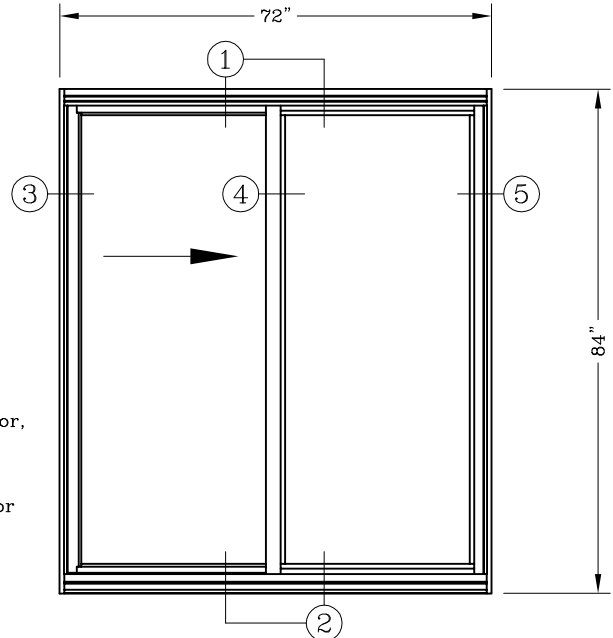
ELEVATION XO Shown 72” x 84” Tested
